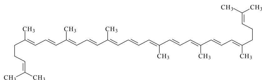
全反式番茄红素化学结构式
