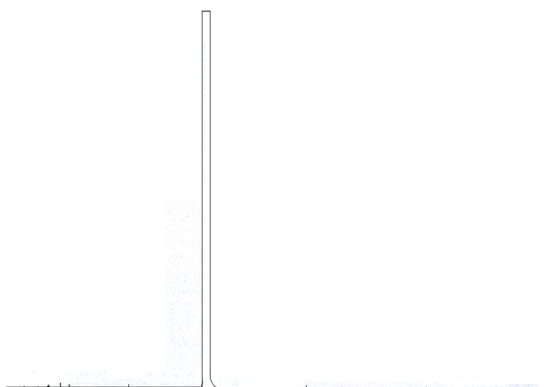
图 B.1 食品添加剂3-甲硫基丙酸乙酯典型气相色谱图
