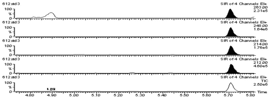
图 A1 氯羟吡啶标准溶液离子色谱图 (10 ng/mL)
