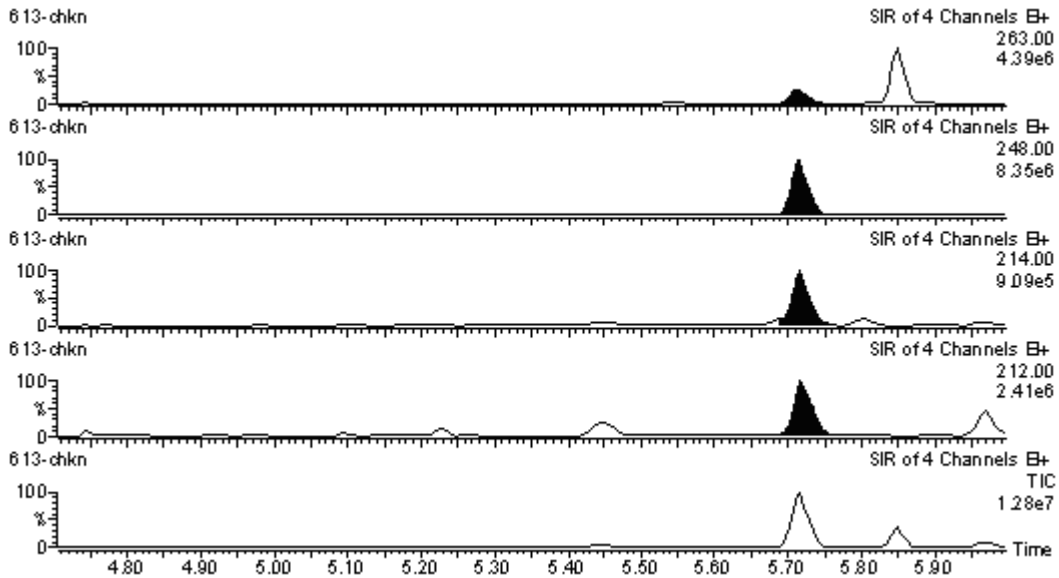
图 A3 鸡肌肉组织空白添加氯羟吡啶试样离子色谱图(10 µg/kg)
