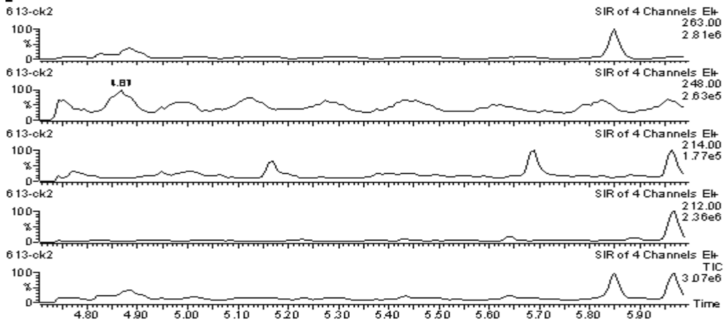
图 A2 鸡肌肉组织空白试样离子色谱图
