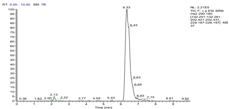
图 A3 猪肝脏组织空白添加呋喃苯烯酸钠试样离子色谱图 (0.5 µg/kg)
