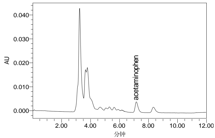
图 A.3 猪肌肉组织空白添加对乙酰氨基酚试样色谱图 (10 µg/kg)
