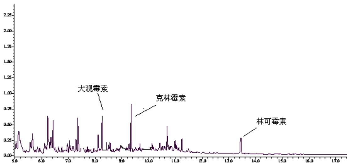
图 A3 猪肌肉组织空白添加林可霉素、克林霉素和大观霉素试样离子色谱图
