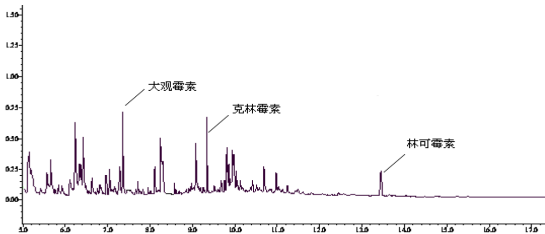
图 A1 标准溶液衍生物离子色谱图
