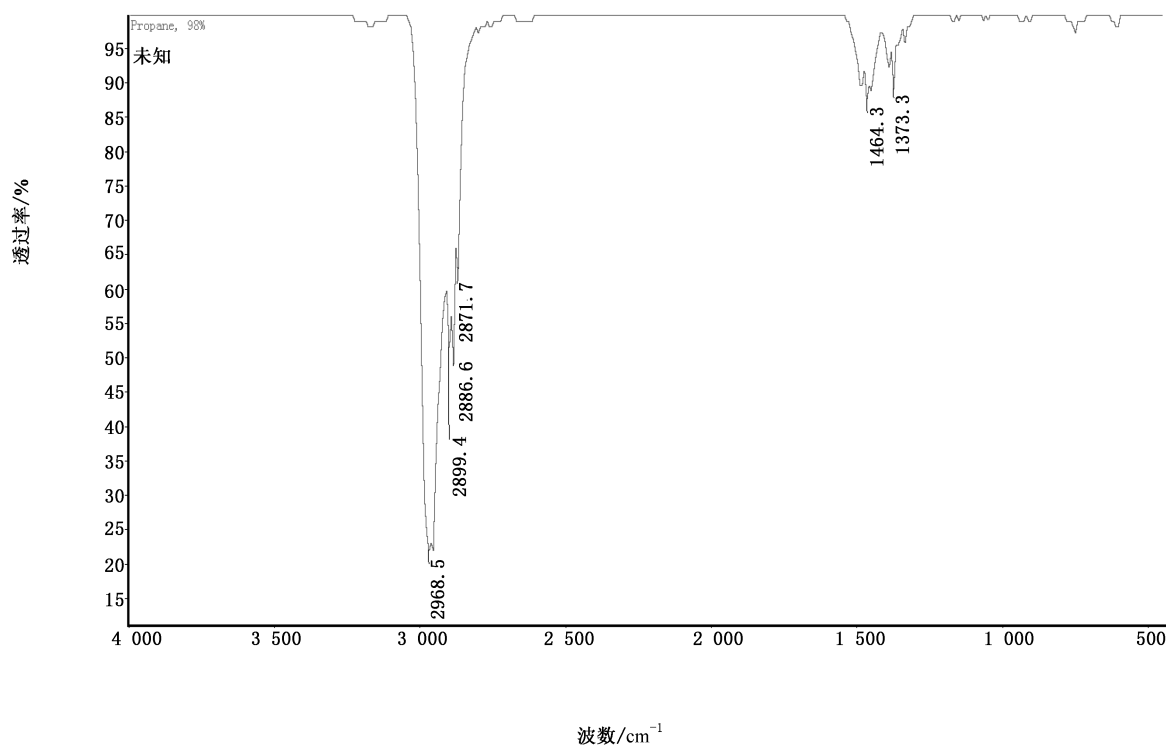
图 B.1 丙烷的红外光谱图
