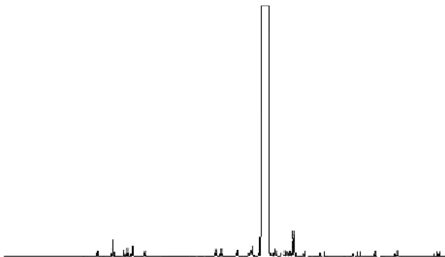
图 B.1 食品添加剂乙酸芳樟酯气相色谱图
