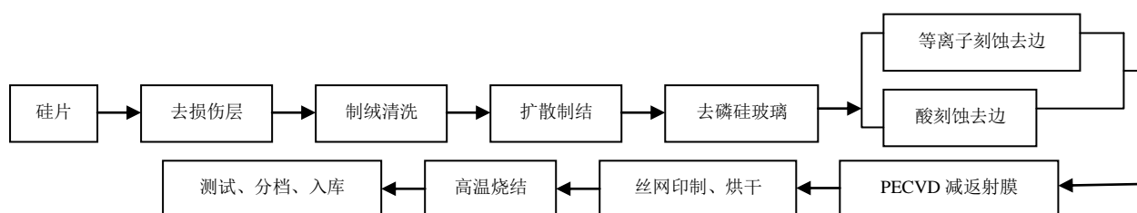
图 A.1 硅太阳能电池片主要生产工艺流程
