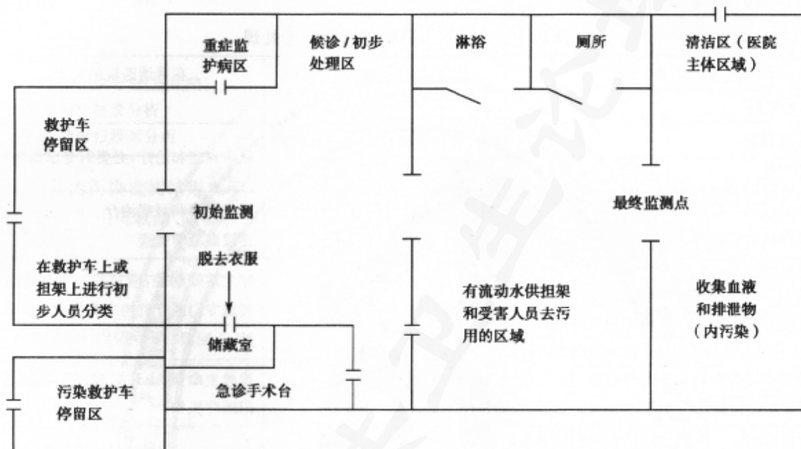
图 D.1 受照人员接收中心规划示意图
