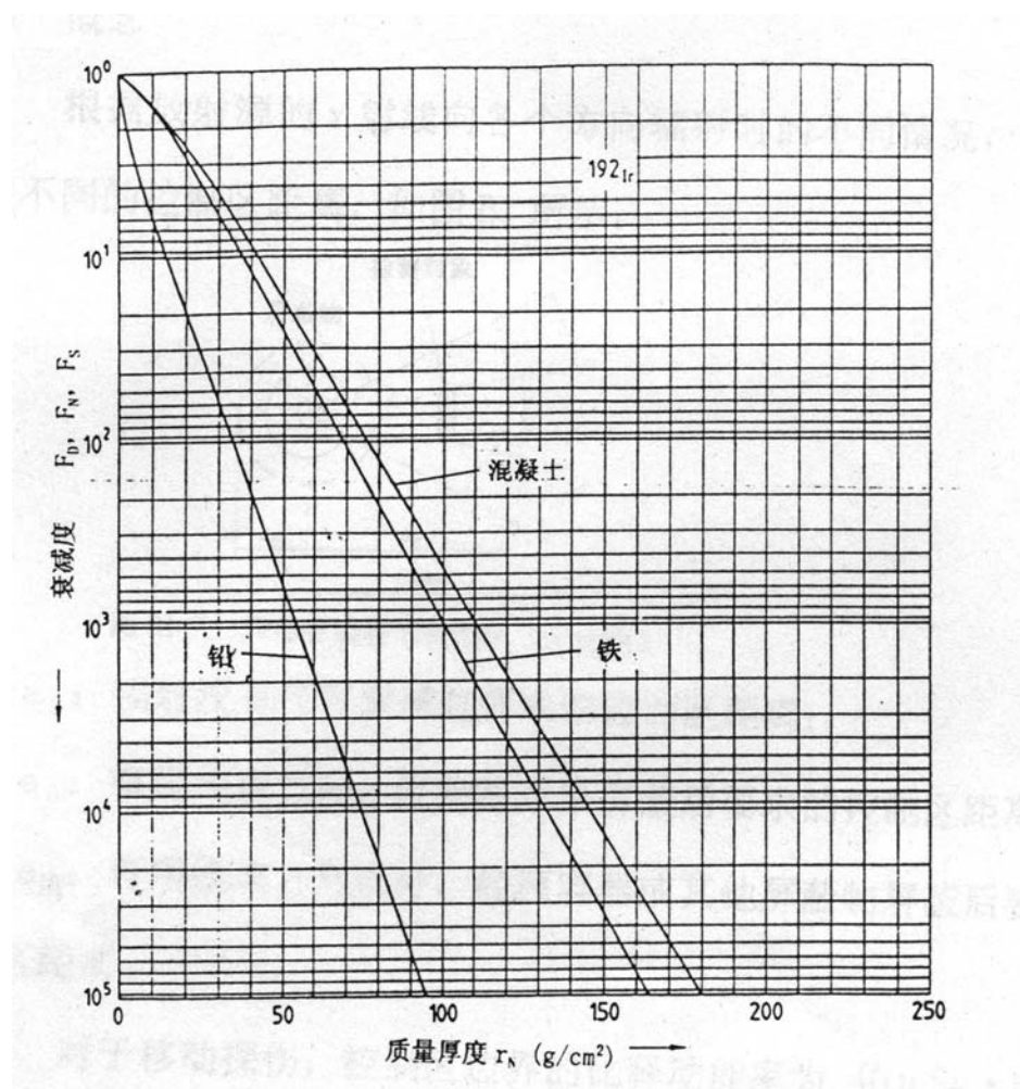
图A2 192 Ir有用线束衰减度为 F_N , 散射线衰减度为 F_S , 泄漏辐射衰减度为 F_0 时不同材料的质量厚度
