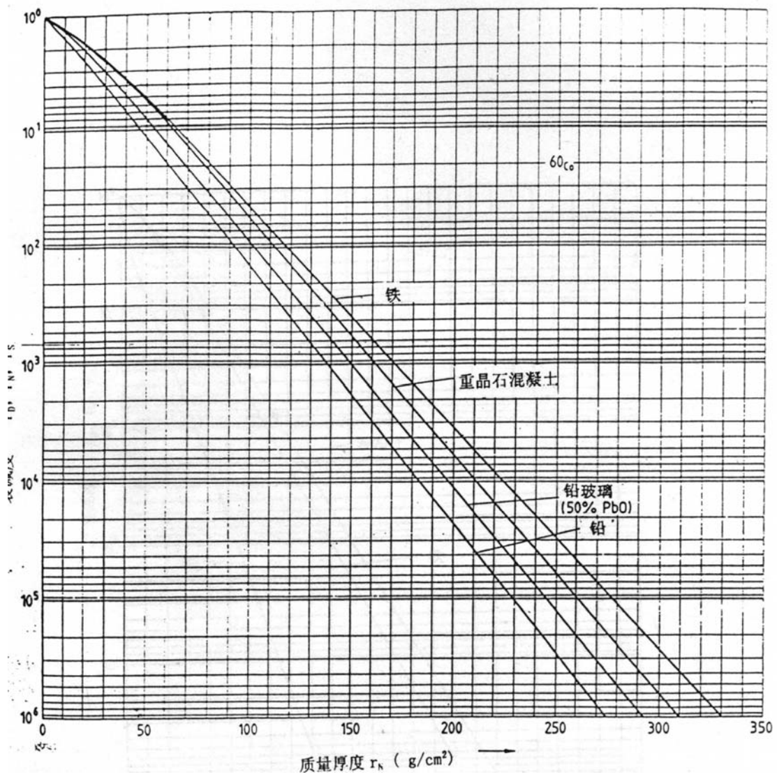
图A1 ^{60}Co 有用线束衰减度为 F_N , 散射线衰减度为 F_s , 泄漏辐射衰减度为 F_D 时不同材料的质量厚度
