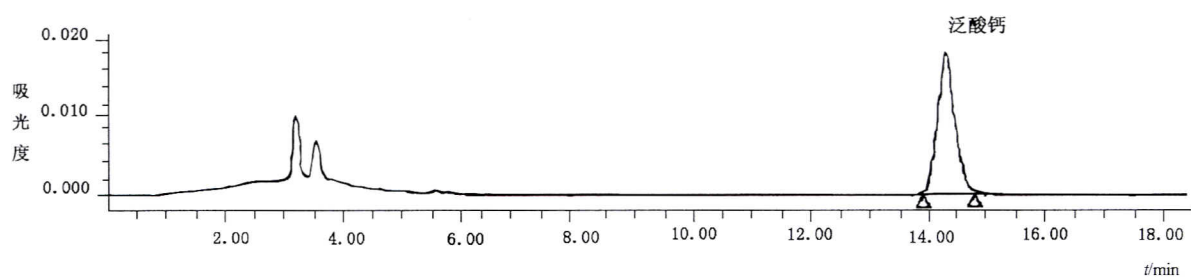
图 1 泛酸钙标准色谱图
