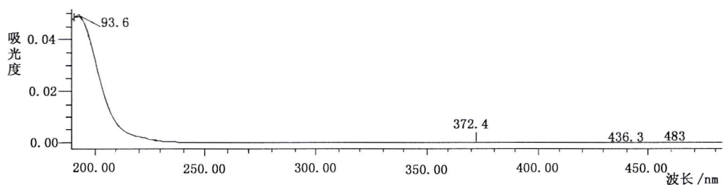
图 3 泛酸钙紫外光谱图
