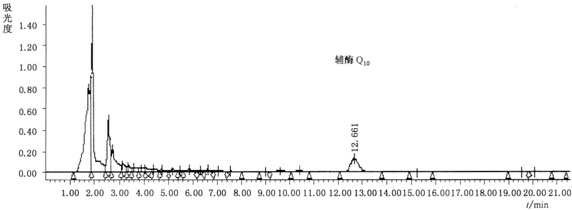
图 2 辅酶 Q 10 试样色谱图
