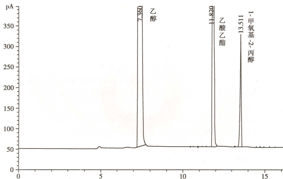
图 1 色谱分离参考图谱
